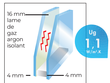
Double vitrage 4 - 16 - 4 ITR + gaz argon
