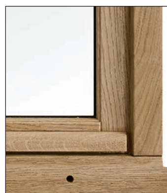
Jet d'eau filant arrondi et drainage rapide
