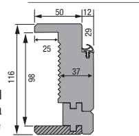
KM1 cloison 98 mm et de 105 à 400 mm
