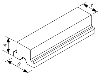
Profilé magnétique
