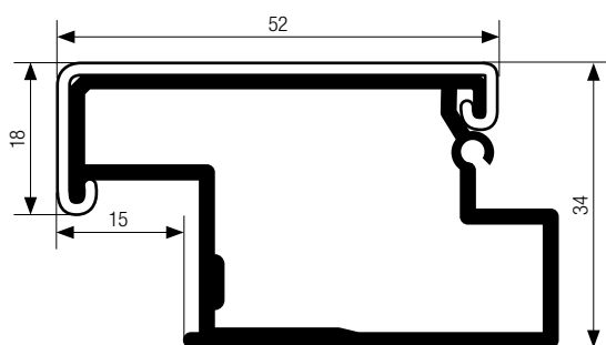
Lame terminale a recouvrement Couvercle Uni 17027591 Partie inf. alu 17799441 Uni+L 17027611 Décor 17021881
