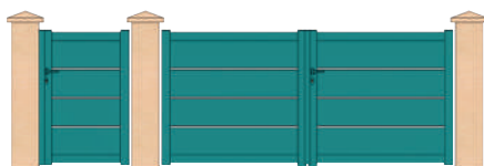
Nanda - RAL 5018 lames horizontales 300 mm + liseré RAL 7035 20 mm
