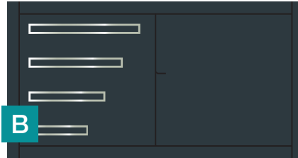
Modèle B : • 1 motif plat évidé : 60 x 2000 mm • 1 motif plat évidé : 60 x 1500 mm • 1 motif plat évidé : 60 x 1000 mm • 1 motif plat évidé : 60 x 500 mm
