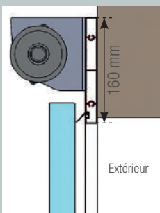
Coupe verticale
